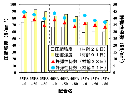
図-2 圧縮強度および静弾性係数試験結果
