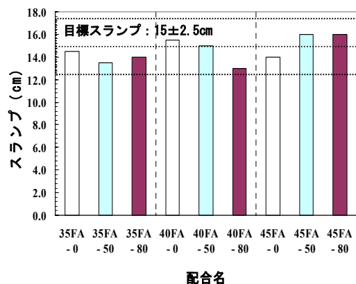
図-1 スランプ試験結果
