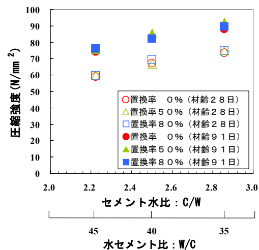
図-3 圧縮強度と水セメント比の関係
