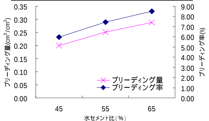
図 - 1 ブリーディング試験結果
