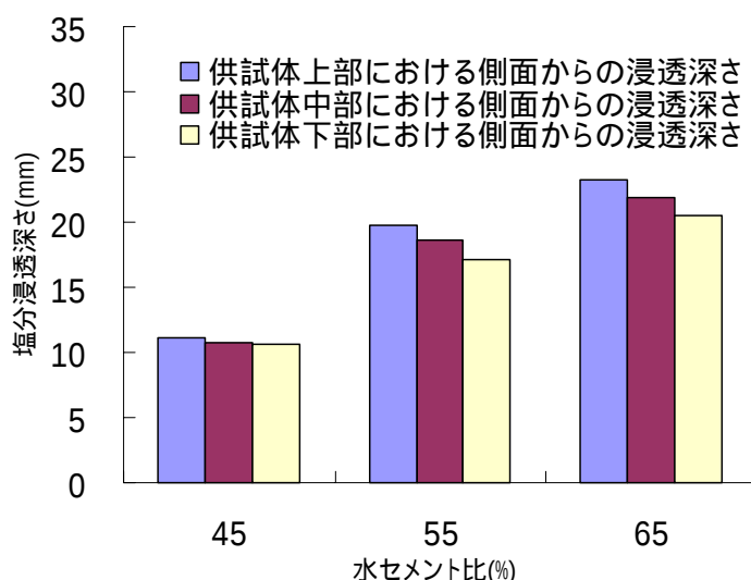
図 - 3 側面方向からの塩分浸透深さ
