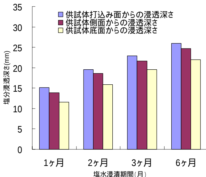
図 - 4 塩分浸透深さと塩水浸漬期間の関係
