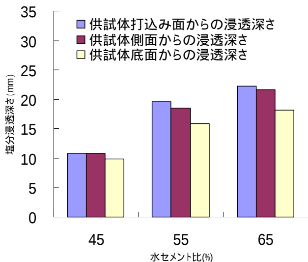
図 - 2 塩分浸透深さの水セメント比による影響
