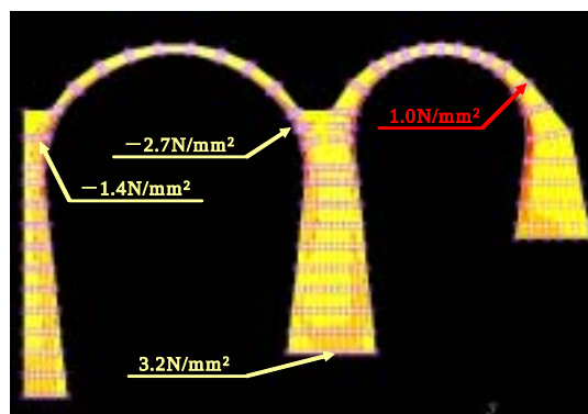
図 3.5 三の沢橋梁における FEM 温度応力練成解析結果
