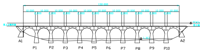
図 2.1③ タウシュベツ川橋梁概略寸法図
