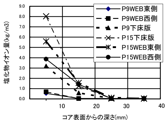
図2-1 浸透塩分量
