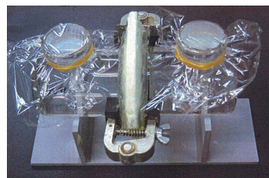
写真4-1 遮塩性試験状況
