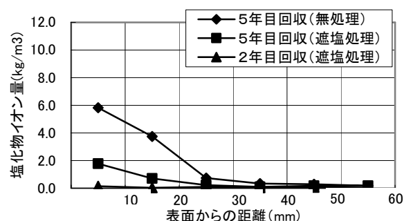
図5-1 P9橋脚暴露試験体浸透塩分量
