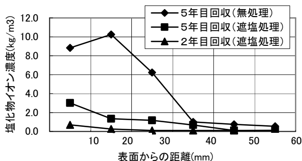
図5-2 P15橋脚暴露試験体浸透塩分量
