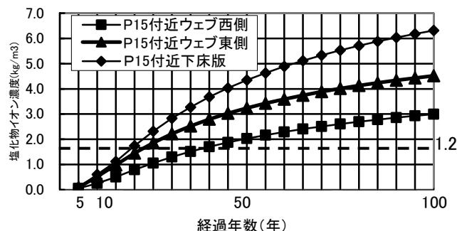
図3-1 塩分量浸透予測
