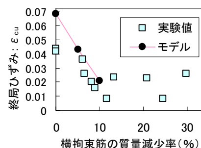
図6 横拘束筋の質量減少率と終局ひずみの関係
