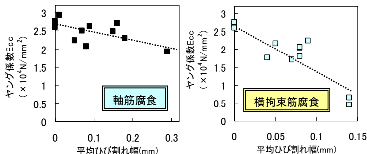
図 4 平均ひび割れ幅とヤング係数の関係
