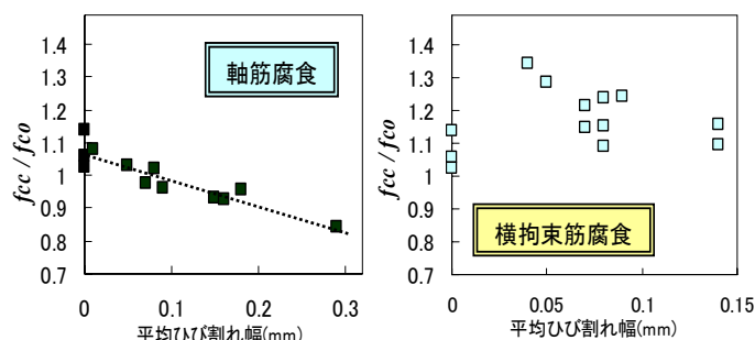
図5 平均ひび割れ幅と最大応力比の関係
