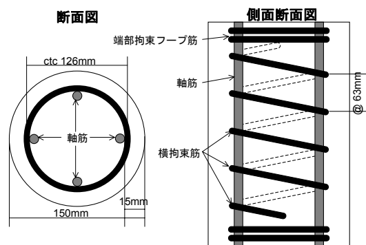
図 1 供試体配筋図
