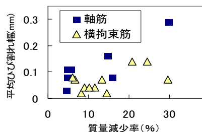
図 2 質量減少率と平均ひび割れ幅の関係
