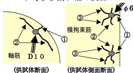
図 3 腐食ひび割れの進展状況
