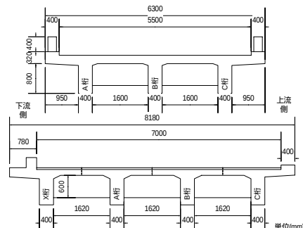
図-1 概略図 (上: A 橋, 下: B 橋)
