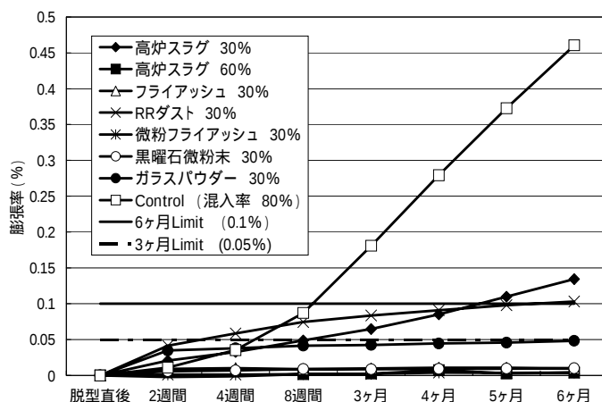
図 3 無機質微粉末混和材の試験結果
