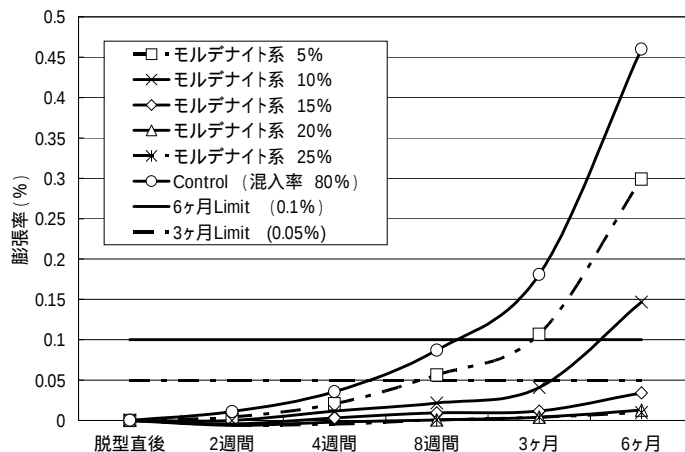
図 2 モルデナイト系ゼオライトの試験結果
