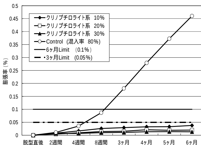
図 1 クリノプチロライト系ゼオライトの試験結果
