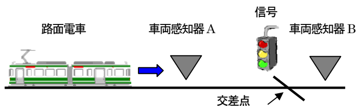
図2: 路面電車と信号、車両感知器の位置関係
