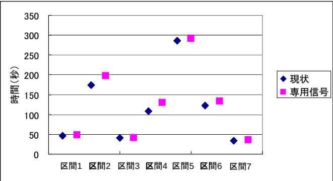
図7： 停止時間
