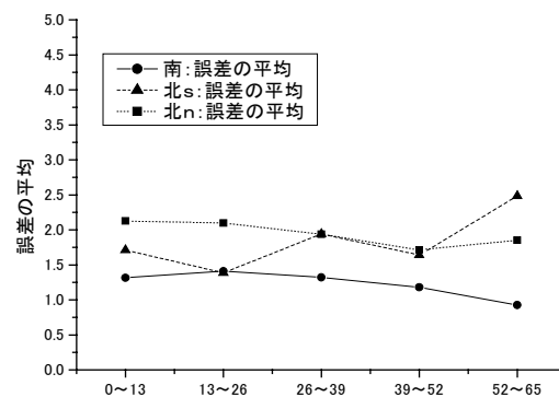
図7 観測角による影響
