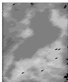
図 1 MODIS による計測温度の画像データ
