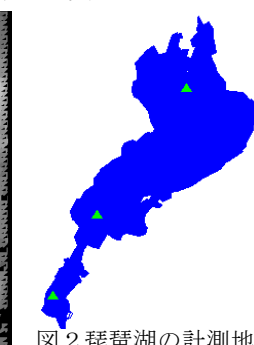
図 2 琵琶湖の計測地点(上から北 n・s 局, 南局)
