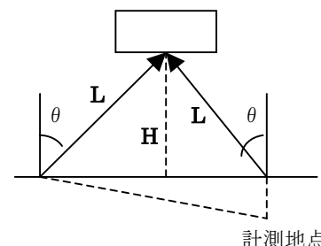
図 3 観測角の取り方
