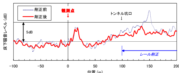
図4 マヤ車床下騒音レベルの変化（近接側軌道）
