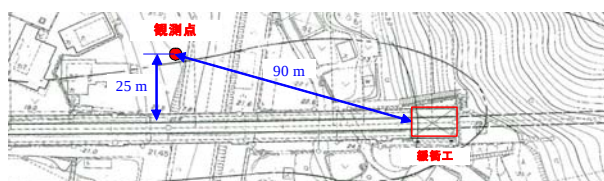
図3 現地平面図
