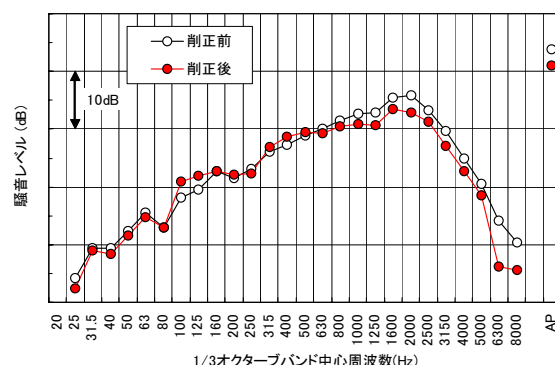
図6 トンネル坑口騒音の周波数スペクトル
