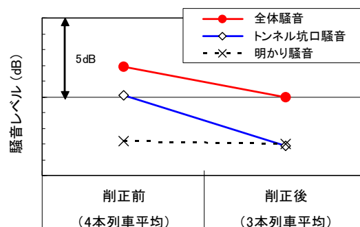
図5 観測点における騒音レベルの変化
