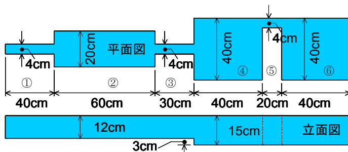
図1 実験装置
