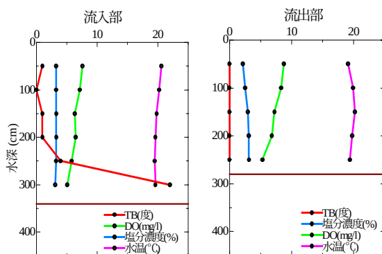
図-3 藻琴湖の流入・流出部の水質
