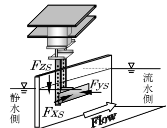
図-3 側壁面に作用する力の測定方法
