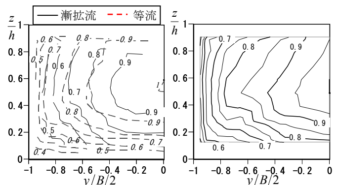
図-5 \bar{B}/\bar{h}=5.9 の漸拡流と等流
