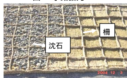
写真-1 粗朶沈床工模型
