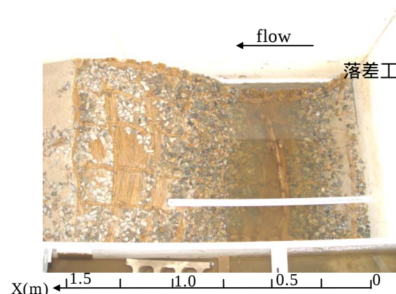
写真-2 粗朶沈床工の被災状況
