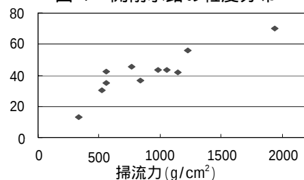
図-8 掃流力と限界粒径の関係
