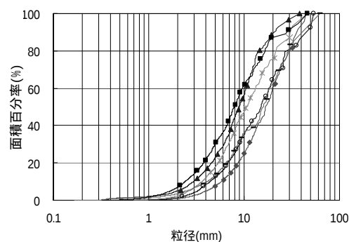
図-7 開削水路の粒度分布
