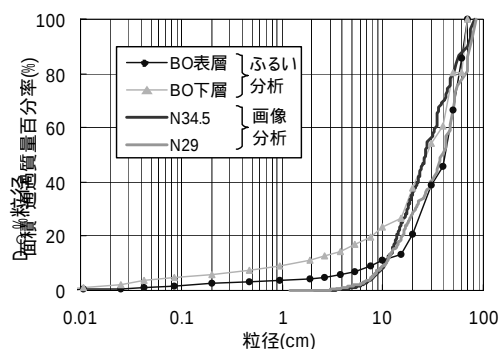
図-9 ふるい分析と画像分析の比較
