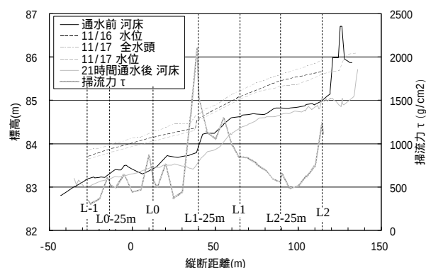
図-6 開削水路の河床高，掃流力等縦断分布
