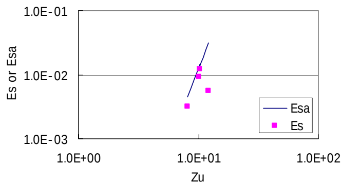
図3 砂の連行係数
