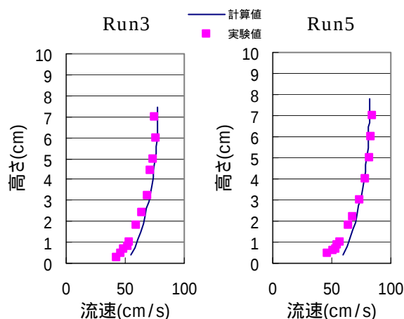
図 1 流速分布の比較
