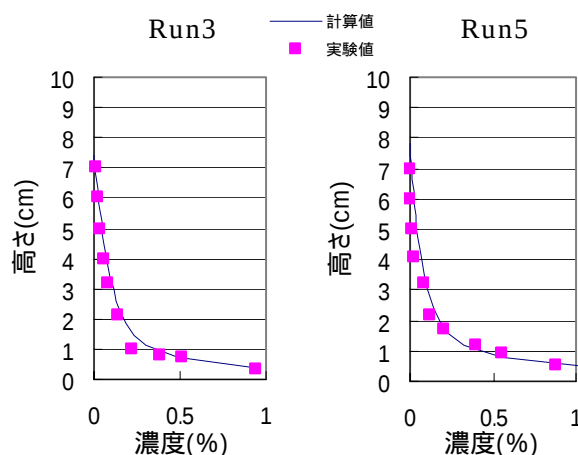
図 2 濃度分布の比較
