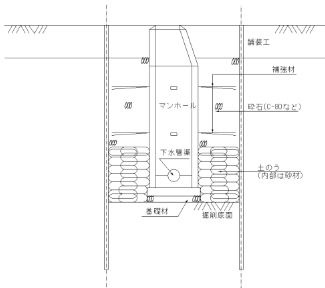
図-2 土のうを利用した浮き上がり対策
