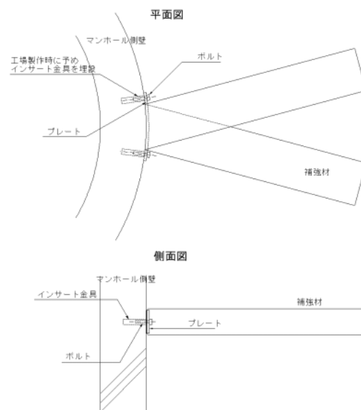
図-3 補強材による浮力への抵抗増加
