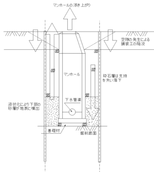
地下鉄の駅舎や共同溝などのボックス構造における代表的な 図-1 マンホールの浮き上がりメカニズム
