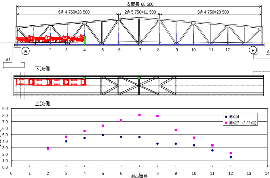
図-2 静的载荷実験の結果
