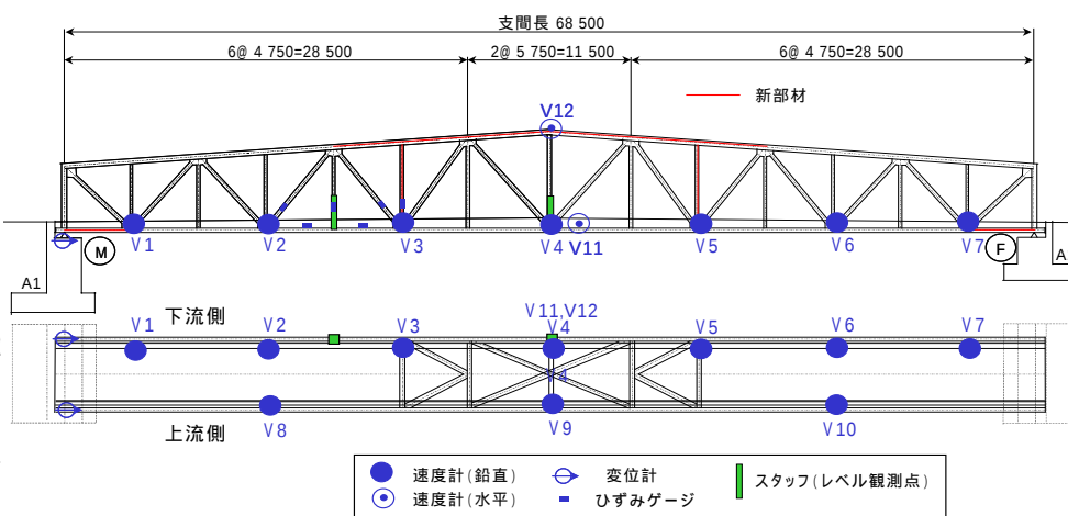
図-1 一般図および測点配置図
