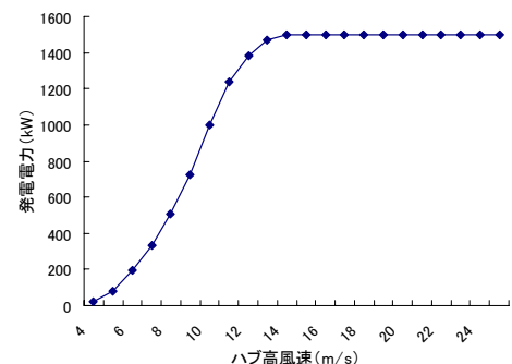
図 1 想定した風車の出力曲線
