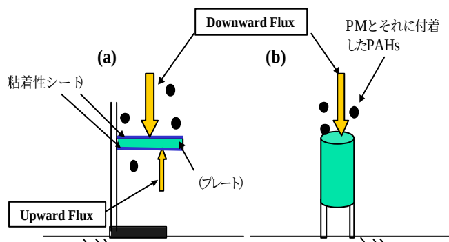
図 1 粘着性表面装置(a)とバケツ状容器(b)
