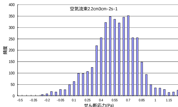
図5 Case1, 空気流束 2.2 \text{ cm}^3 \text{ cm}^{-2} \text{ s}^{-1} ヒストグラム
