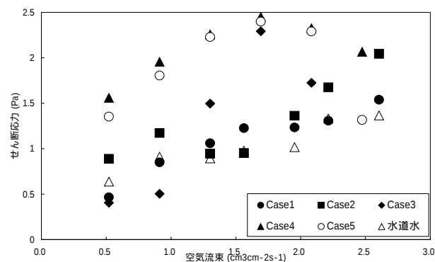
図7 \tau_{3\sigma} と空気流束の関係図
