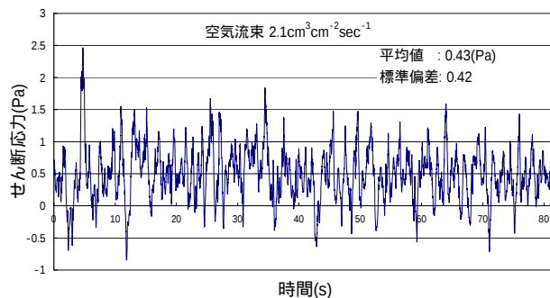
図4 せん断応力経時変化(Case3)
