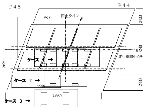
図-2 荷重車による載荷位置図
