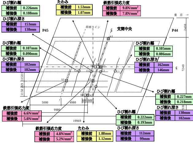
図－3 実橋載荷試験の計測結果
