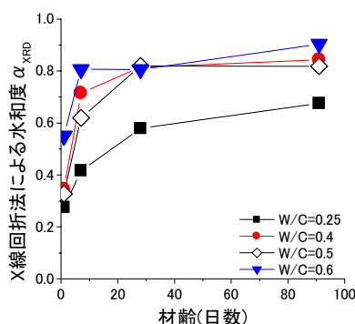
図-2 X線回折法による水和度
