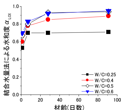
図-1 結合水量法による水和度
