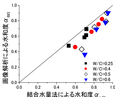
図-5 画像解析法 VS.結合水量法
