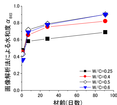
図-3 画像解析法による水和度
