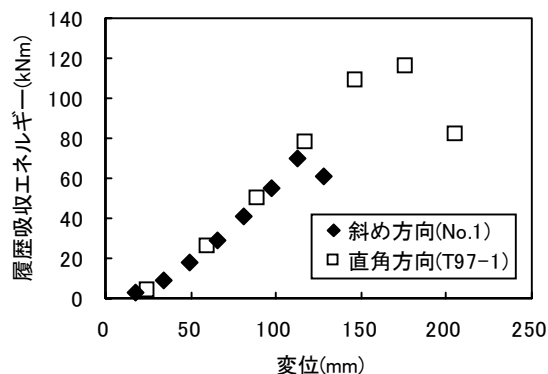
図5 変位と履歴吸収エネルギーの関係
