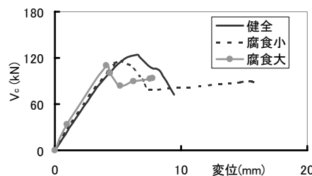
図 4 V_c -変位関係
