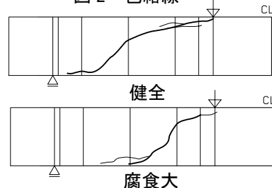
図 3 ひび割れ状況
