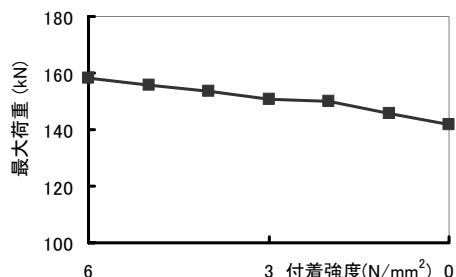
図6 付着性能低下の影響
