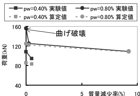
図10 既往の結果と算定値の比較
