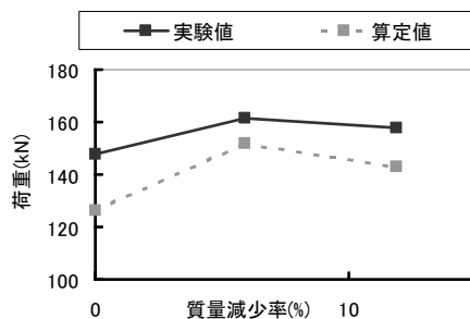
図9 実験値と算定値の比較
