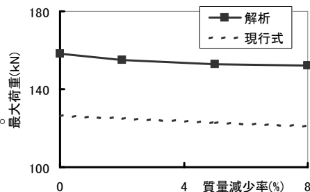
図5 引張性能低下の影響
