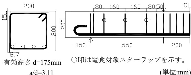
図 1 供試体形状・寸法
