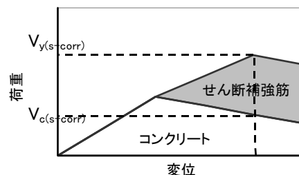
図7 付着性能低下による V_c 低下
