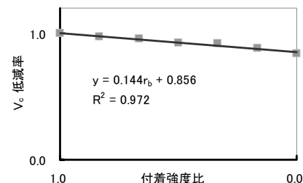
図8 V_c 低減率-付着強度比関係
