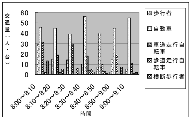
図 - 1 10分間隔の交通量
