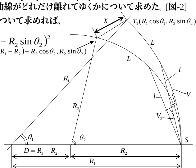
[図-2] Xの算出根拠略図
