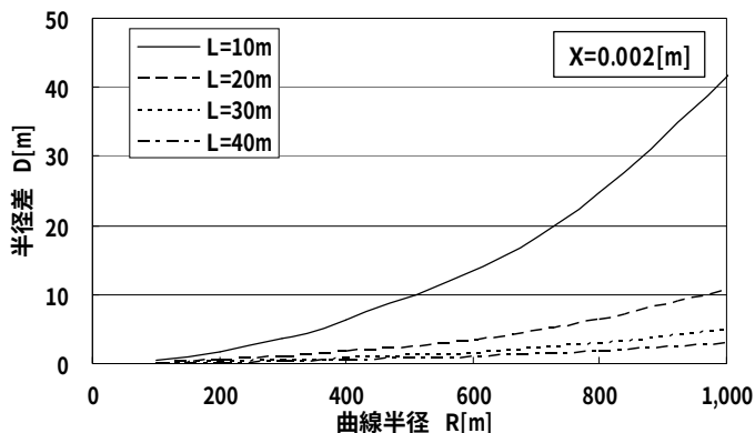
[図-4] (d)式で、 R の変化に対する D の変化( X=0.002\text{m} )
