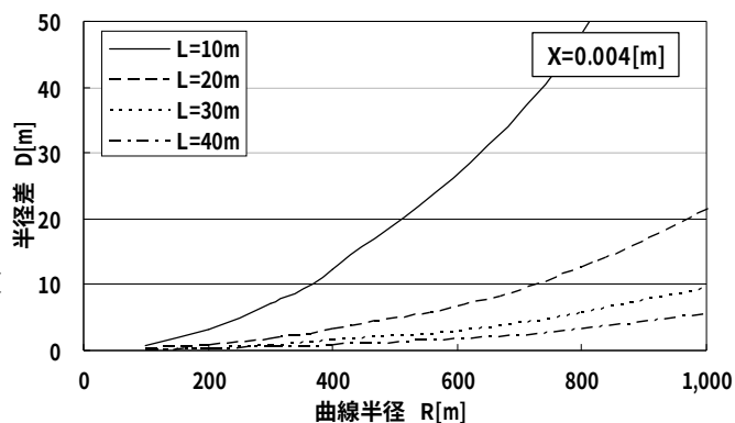
[図-3] (d)式で、 R の変化に対する D の変化( X=0.004\text{m} )
