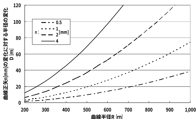
[図-1] 曲線正矢+ n[\text{mm}] の変化に対する半径の変化
