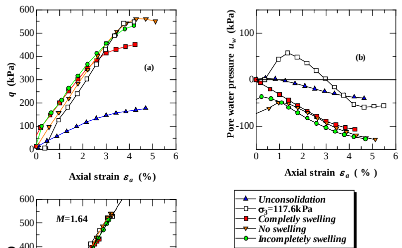
図-2 カタルボ試料を用いた試験結果
