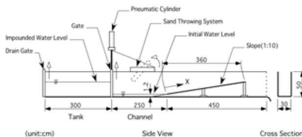
図-1 実験装置
