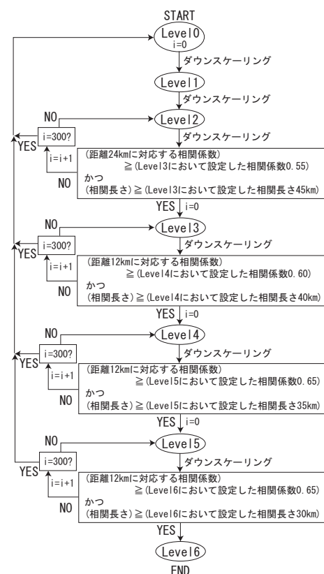
図1：空間相関の導入プロセス
