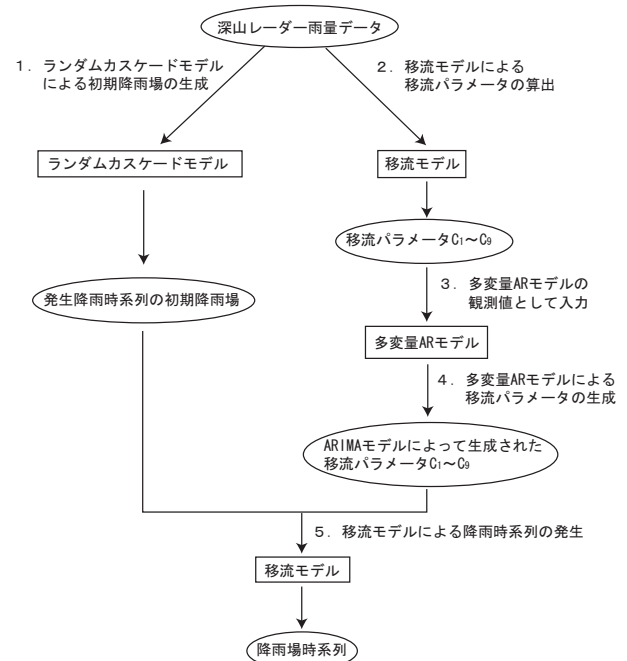
図3：降雨場時系列発生プロセス
