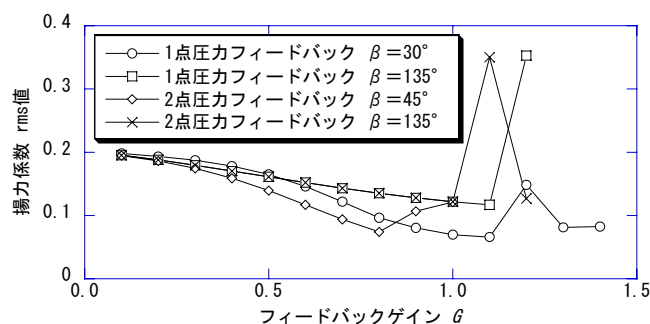
図-4 ゲインの違いによる揚力係数 rms 値の変化
