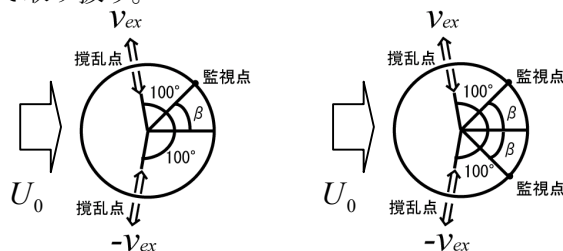
(a) 1点圧力フィードバック (b) 2点圧力フィードバック
