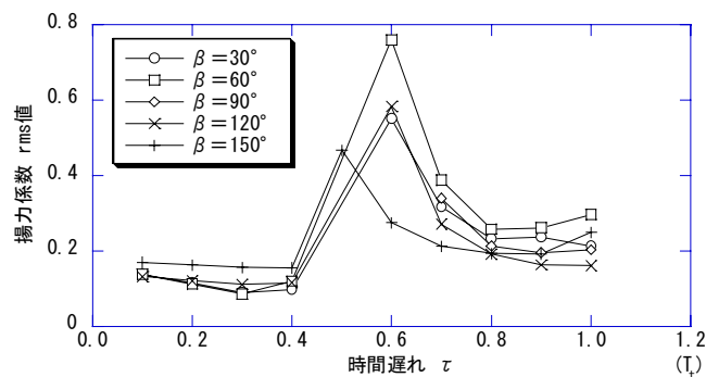
図-3 時間遅れの違いによる揚力係数 rms 値の変化 ( G=1.0 に固定、2 点圧力フィードバック)
