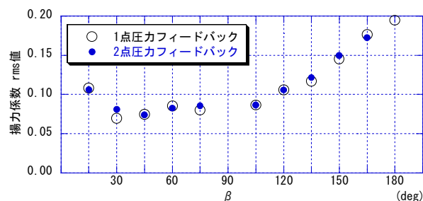
図-5 各監視点で最も制御効果が高かったときの揚力係数 rms 値の変化
