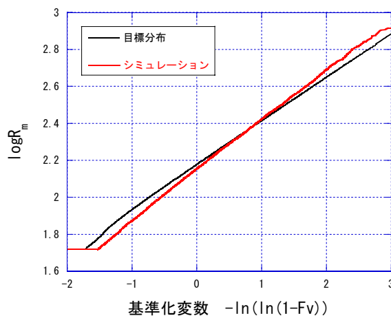
図1 Vickery手法による R_m の確率分布
