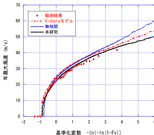
図3 千葉における上空風の年最大風速
