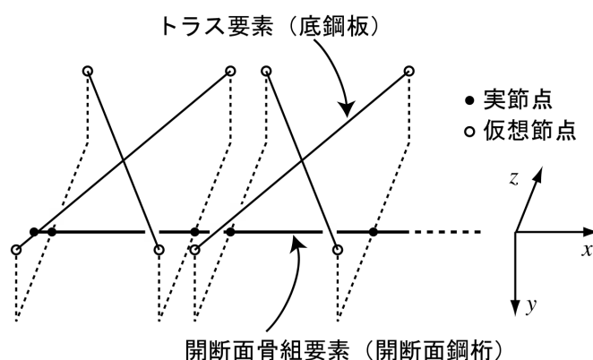
図-2 骨組構造解析の全体モデル
