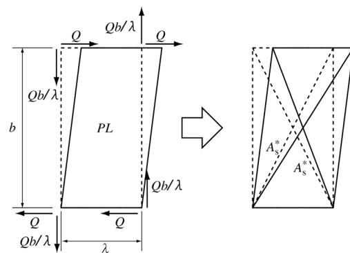
図－3 セン断を受ける鋼板のトラス換算
