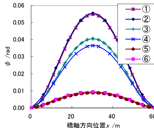
図－4 ねじれ角の橋軸方向分布
