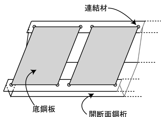
図-1 鋼逆 \pi 形合成桁橋架設時の構造
