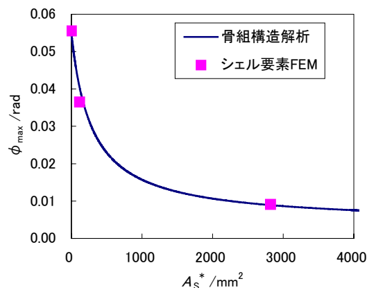
図－5 トラス換算断面積の影響
