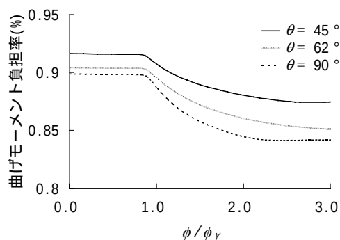
Fig.3 面内回転角とフランジによる曲げ負担率の関係
