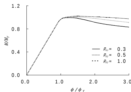
Fig.5 面内回転角と曲げ強度の関係 ( \gamma_{fl}^*=1.0 )
