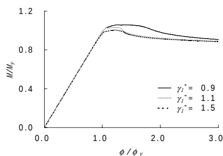
Fig.4 面内回転角と曲げ強度の関係 ( R_{fl}=0.5 )
