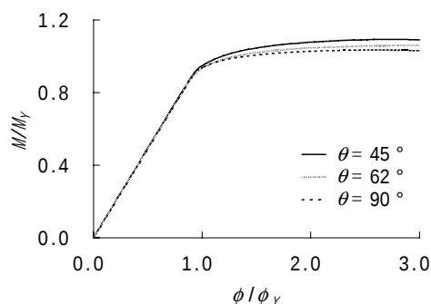
Fig.2 面内回転角と曲げ強度の関係
