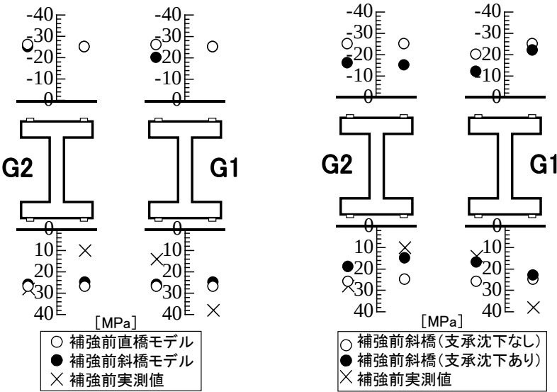
図-5 斜角の影響
