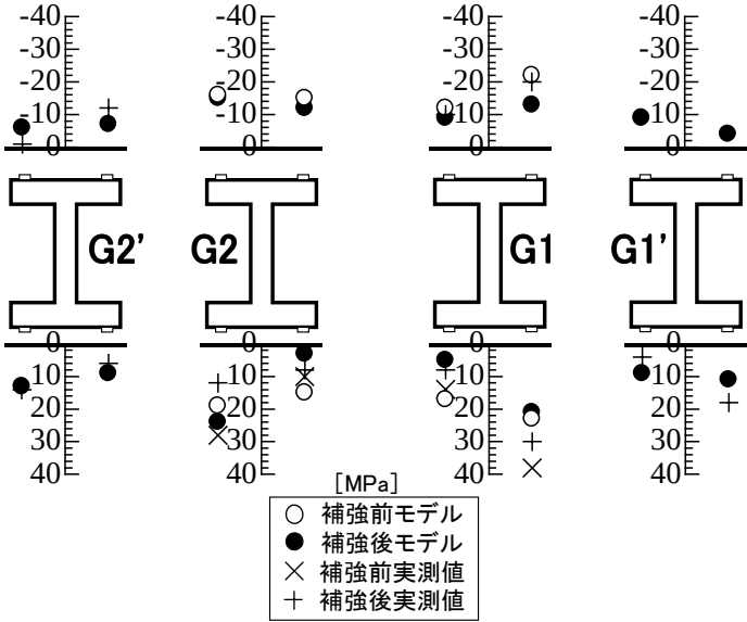
図-7 補強前後の解析値と実測値
