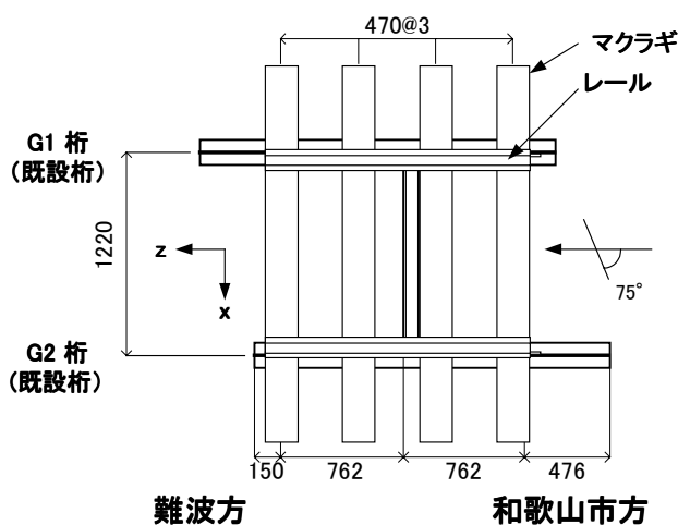
図-1 補強前の橋梁平面図
