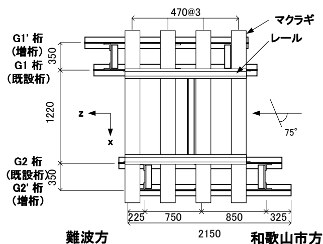
図-3 補強後の橋梁平面図
