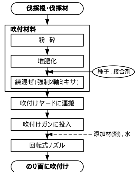
図-1 『根をリサイクル工法』施工フロー図
