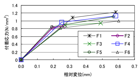
図-3 付着構成則（付着応力-相対変位）
