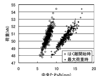
図-6 荷重-中央たわみ関係
