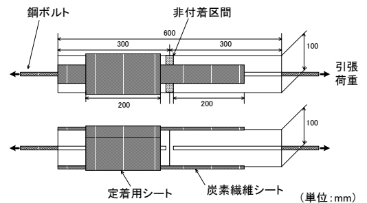
図-1 曲げ載荷試験供試体概要
