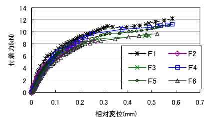
図-2 付着力-相対変位（試験結果）
