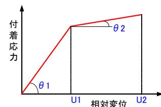
図-5 不確定性を考慮した付着構成則
