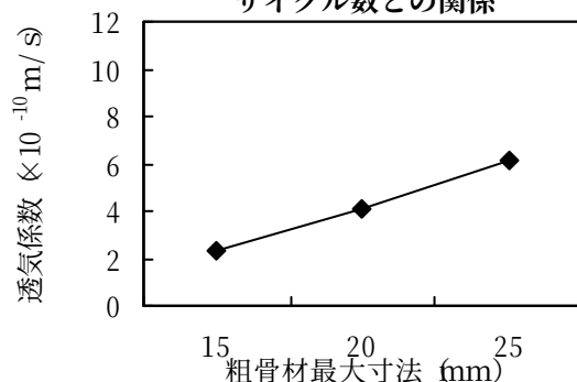
図-5 透気係数と粗骨材の最大寸法との関係
