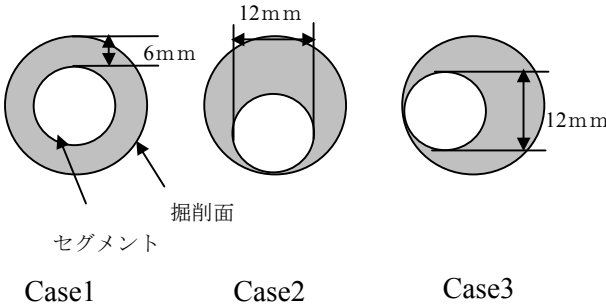
図5 後続沈下における解析ケース
