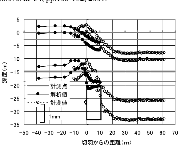
図4 トンネル縦断方向鉛直変位図
