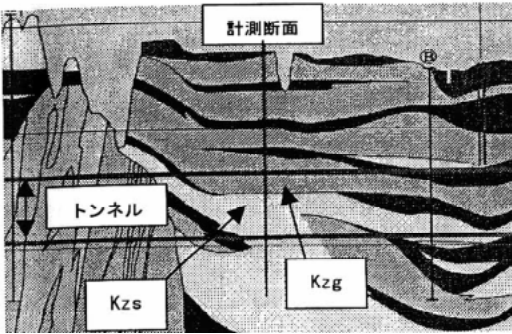
図1 地質縦断面図
