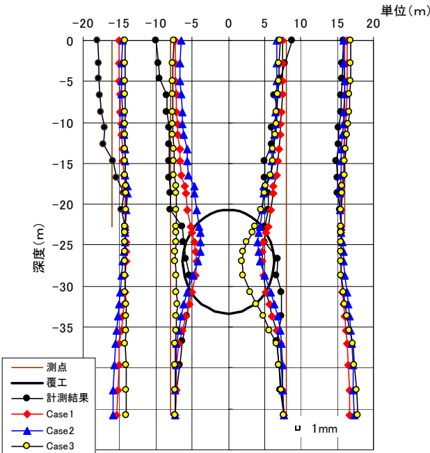
図6 横断面水平変位
