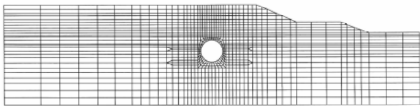
図2 二次元解析モデル
