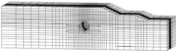
図3 三次元解析モデル
