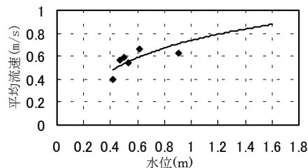
図-4 水位と平均流速の関係
