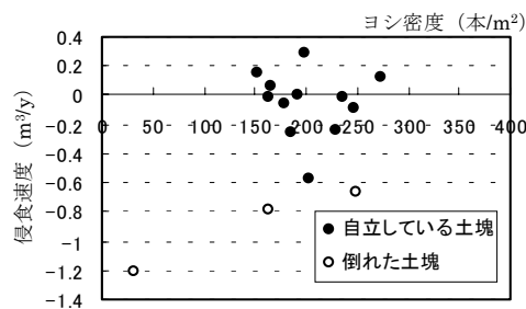
図-9 土塊の侵食速度
