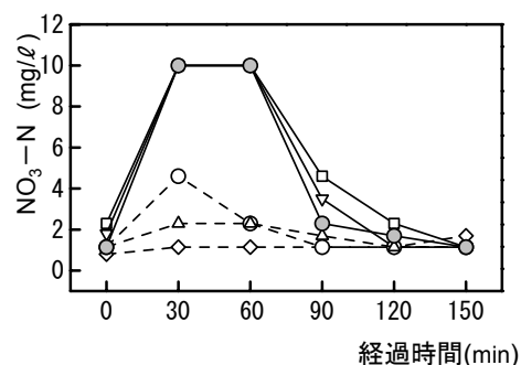
(b) 浸出水における硝酸態窒素の変動
