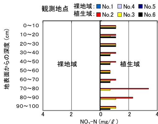
図-3 土壌の含有する硝酸態窒素の鉛直分布
