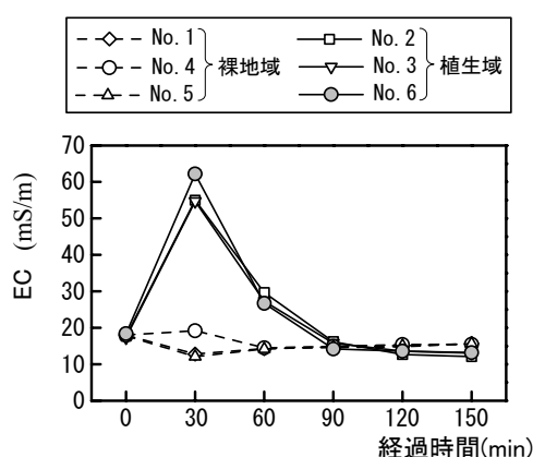
(a) 浸出水における EC の変動
