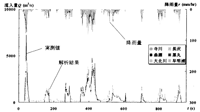
図-5 早明浦ダム流入量の実測値と計算値
