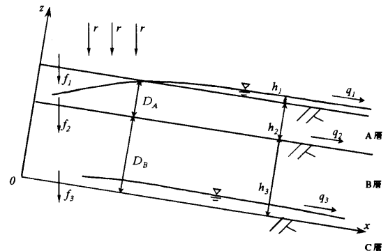
図-2 斜面における土層および降雨流出モデル
