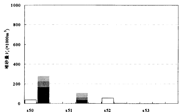
図-7 堆砂量の実測値と計算値（大橋ダム）
