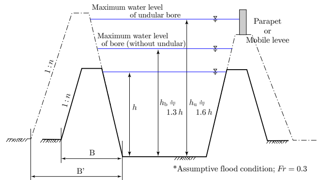
図-5 洪水時に段波が発生した場合の水深と堤防高の関係（H.W.L. に達するような洪水時に段波が発生すると、多くの場合、設定されている余裕高だけではその段波を河道内に留めることは難しい。また、波状性により波高はこれを無視した場合の波高に比べて 20%以上も大きくなることから波状性を考慮した上で検討を進めるべきである）
