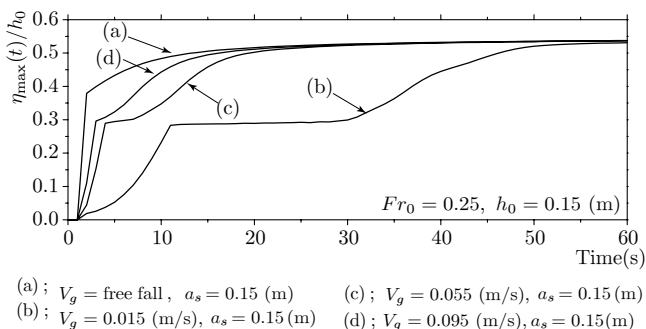
図-3 ゲートの閉鎖法の違いによる最大波高の時間的変化の差異（いずれの閉鎖方法であっても最終的には同じ波高にまで到達する）
