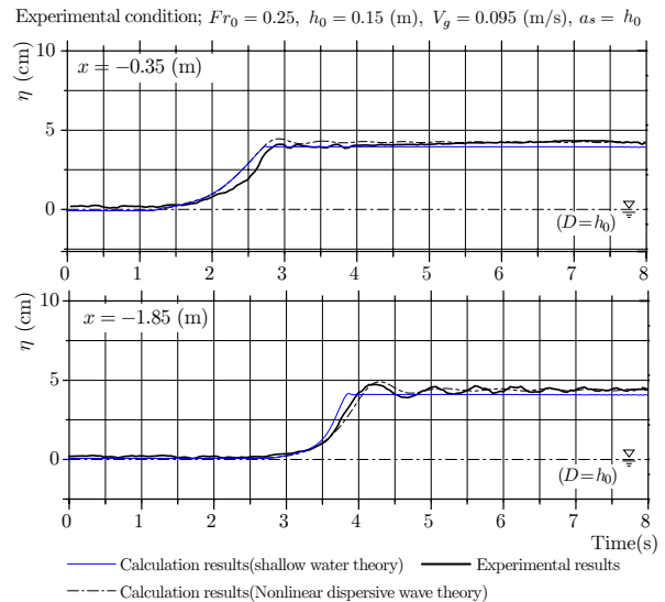
(a) ゲートを緩閉した場合
