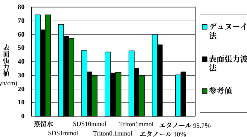
図-5 実験結果
