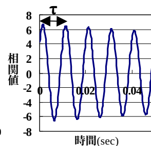
図-4 相互相関関数
