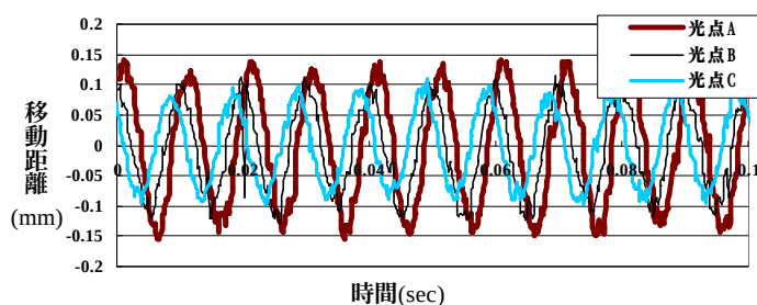
図-2 SDS(1mmol)の光点の移動距離と時間の関係
