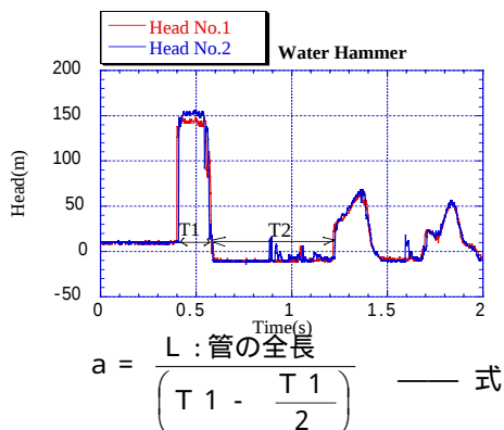
図6 負圧部伝播速度の求め方
