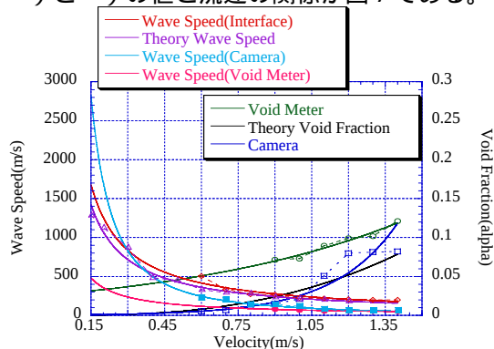
図7 流速と負圧部伝播速度の関係
