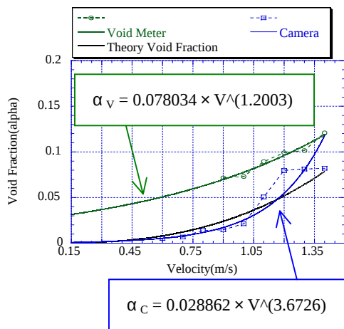
図5 各流速とボイド率の関係
