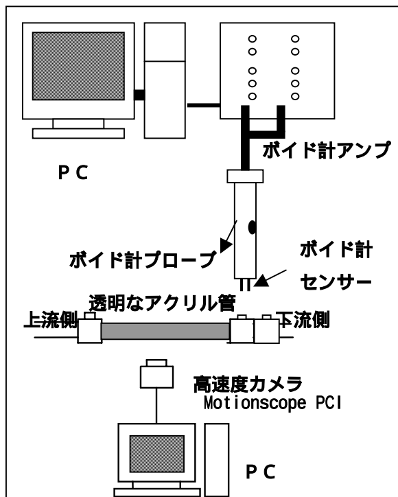
図 1 気泡計測用装置
