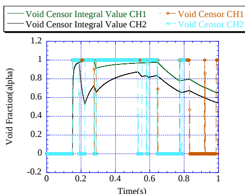
図 3 ボイド率の時間変化(流速約 1.4m/s)
