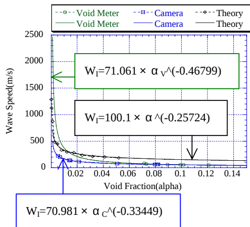
図8 負圧部伝播速度とボイド率の関係
