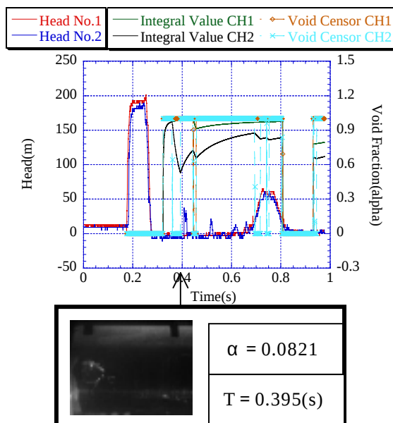
図4 水撃波形にプロットしたボイド率
