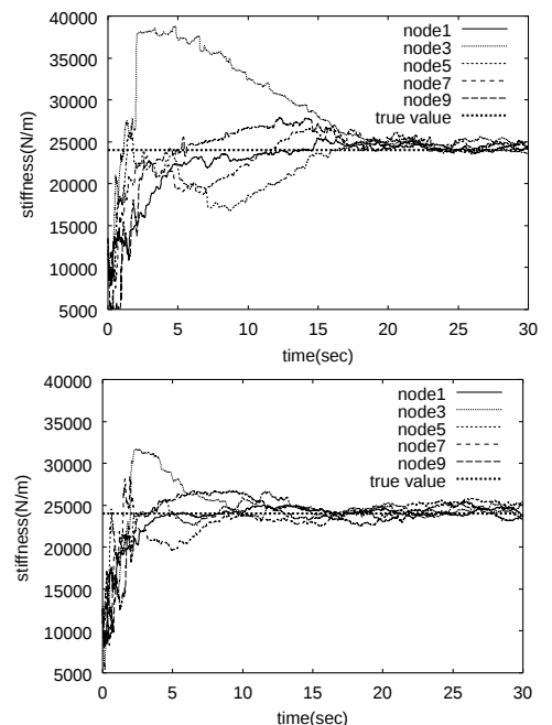
図-2 剛性の同定結果のフィルタ粒子の平均値の時刻歴 (上: CASE1, 下: CASE2)
