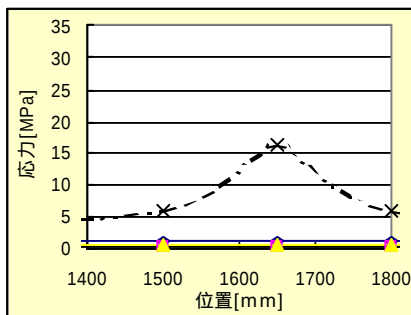
図6. 無限長さ梁の曲げ応力度
