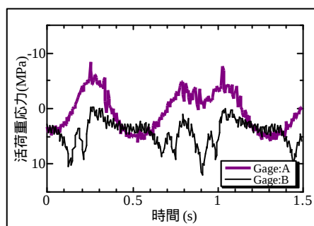
図4. 橋軸方向における応力の比較
