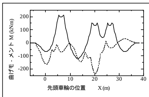
図2. 桁に作用する曲げモーメント
