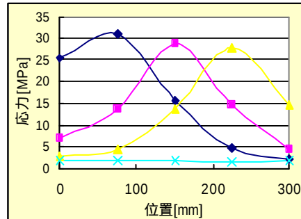
図7. 半無限長さ梁の曲げ応力度
