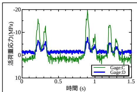
図5. 橋軸直角方向における応力の比較
