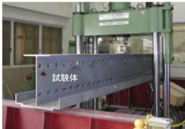
写真-1 試験体および荷重状況
