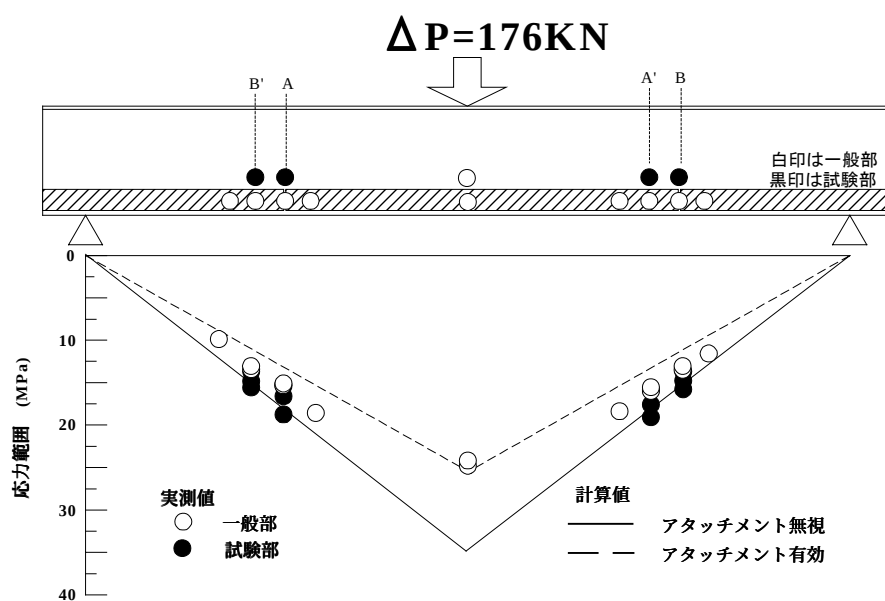
図-1 試験体長手方向の応力分布（全体）
