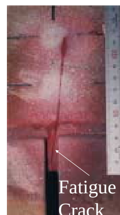
写真-3 進展中の疲労亀裂(2 体目)
