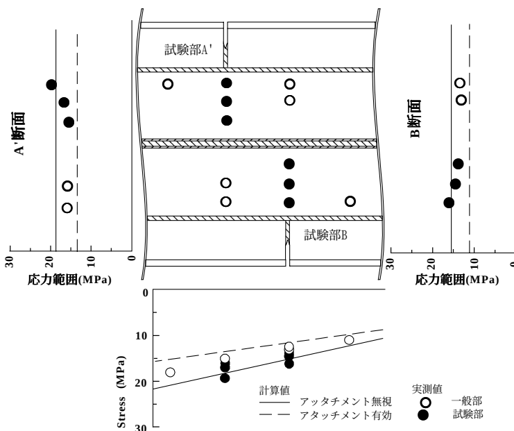
図-2 A',B 断面の応力分布
