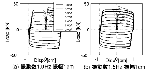
図4 正弦波加振試験
