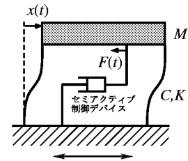
図1 擬似負剛性制御の例
