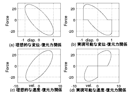
図2 負剛性および擬似負剛性の荷重応答特性
