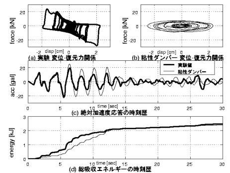
図6 一自由度モデルでの効果の検証
