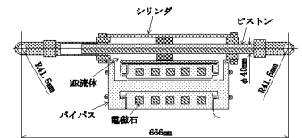
図3 MR ダンパー
