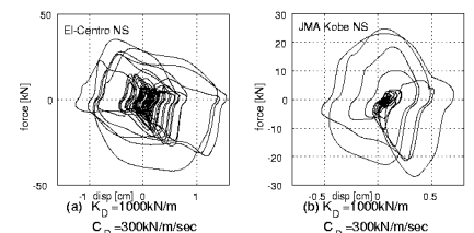
図7 固有周期 1.14sec のモデルの
