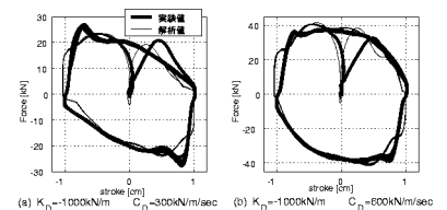
図5 擬似負剛性の履歴の実現
