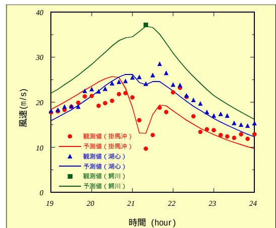
図3 平均風速の観測値と予測値との比較
